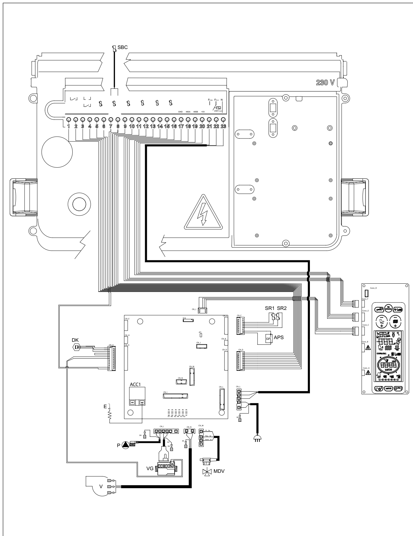
Рис. 20 Електрична схема RBTFS
