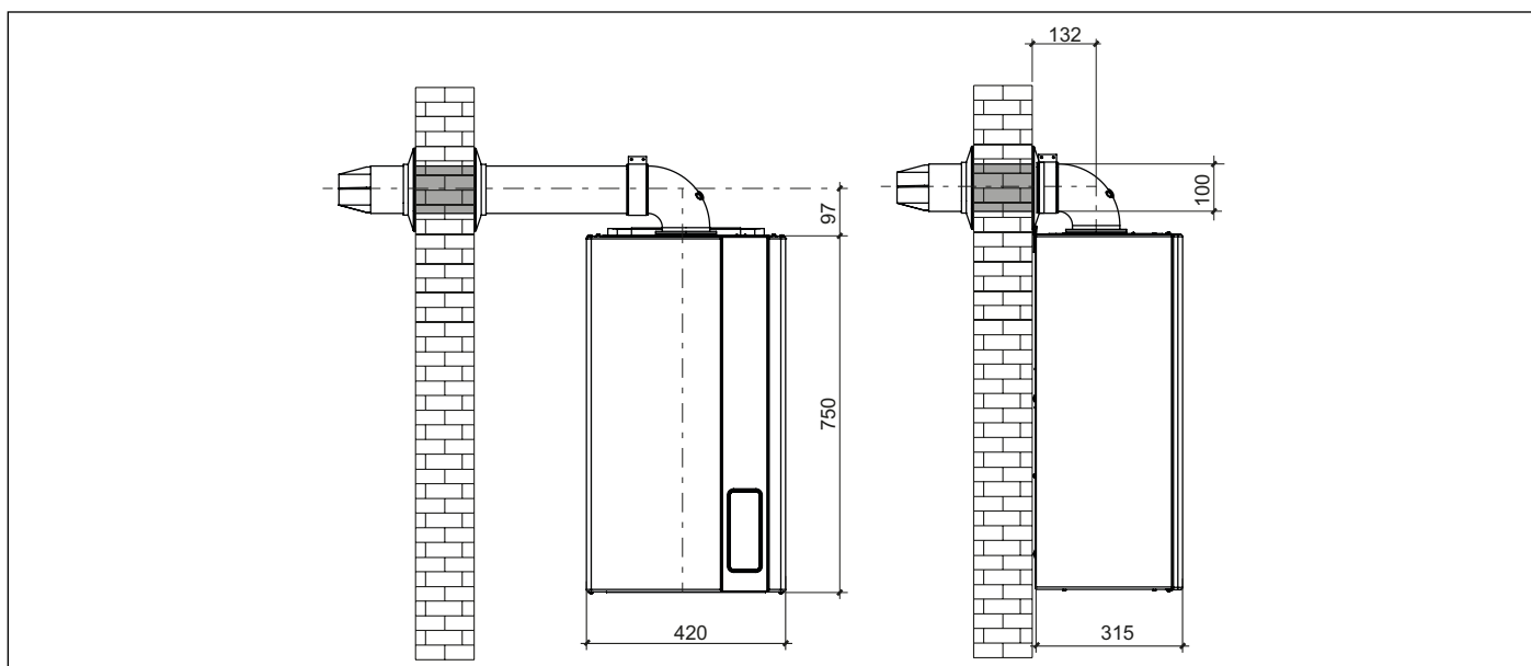
Рис. 12 Розміри для підключення до коаксиальної системи забору повітря/викиду продуктів згоряння
