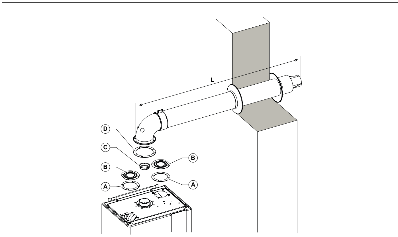
Рис. 11 Забор повітря та викид продуктів згоряння за допомогою коаксиальних труб
