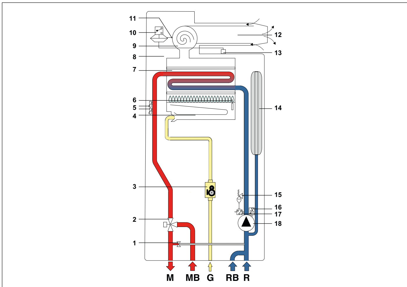
Рис. 7 Схеми гідравлічних підключень RBTFS
