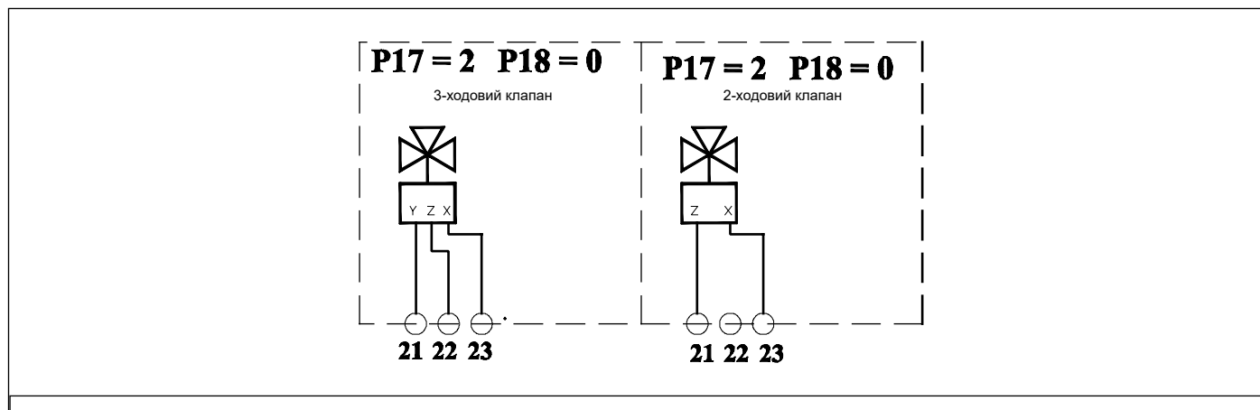
Рис. 29 Схема підключення багатфункційного реле (X = загальний; Y = на котел; Z = на колектор)
