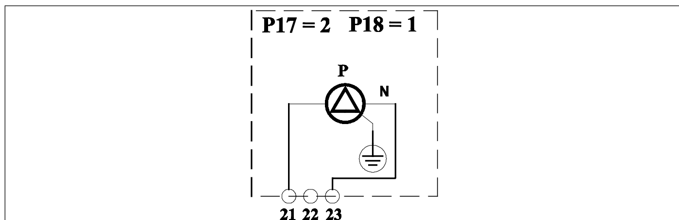
Рис. 23 Схема підключення багатфункційного реле
