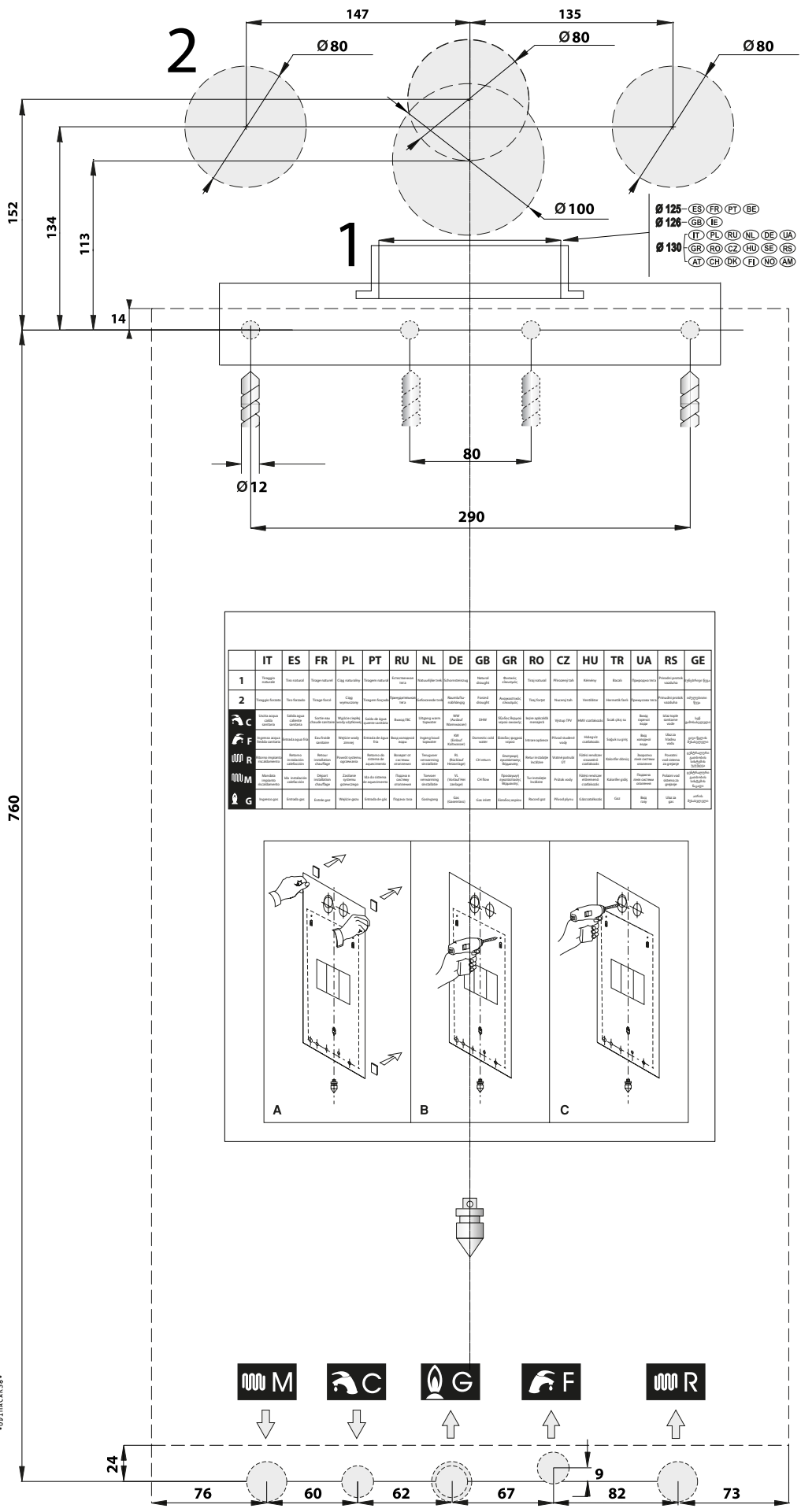
Рис. 9 Паперовий шаблон.
