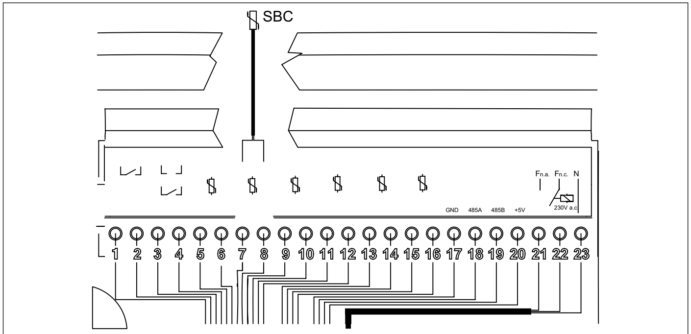
Рис. 21 Докладна електрична схема RBTFS
