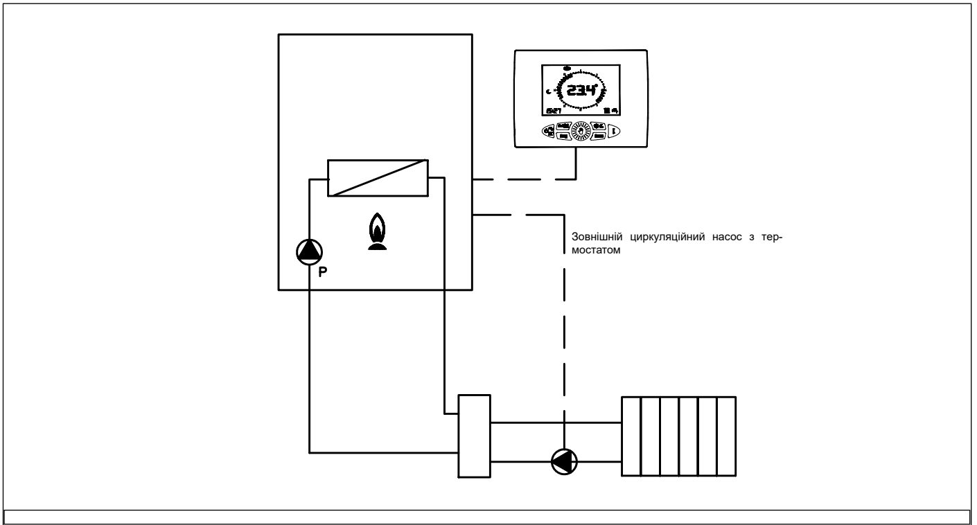
Рис. 32 Робота реле по зовнішньому запросу (P17=1)
