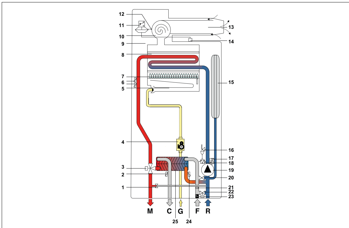
Рис. 8 Схеми гідравлічних підключень CTFS
