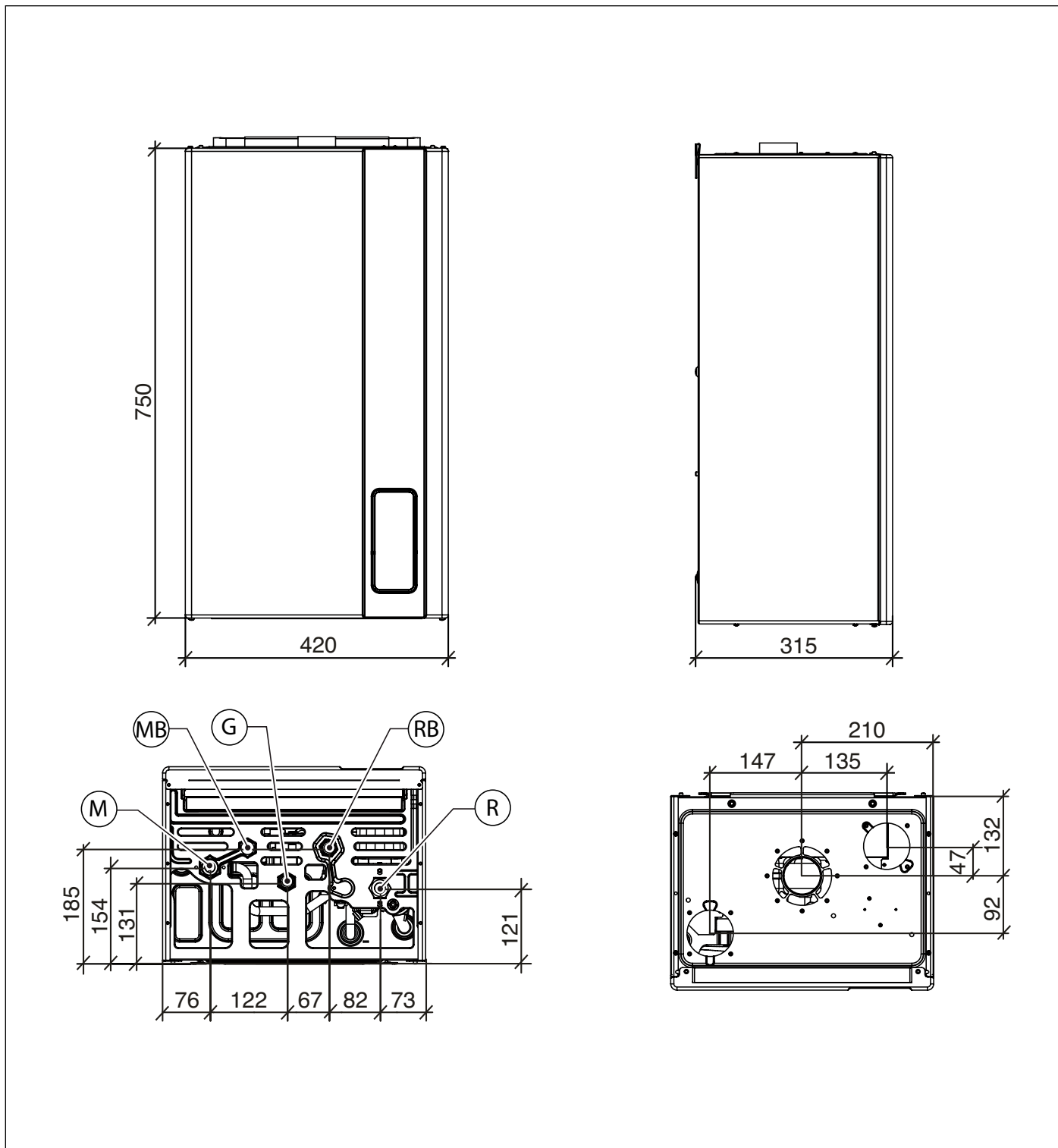
Рис. 5 Габарити RBTFS
