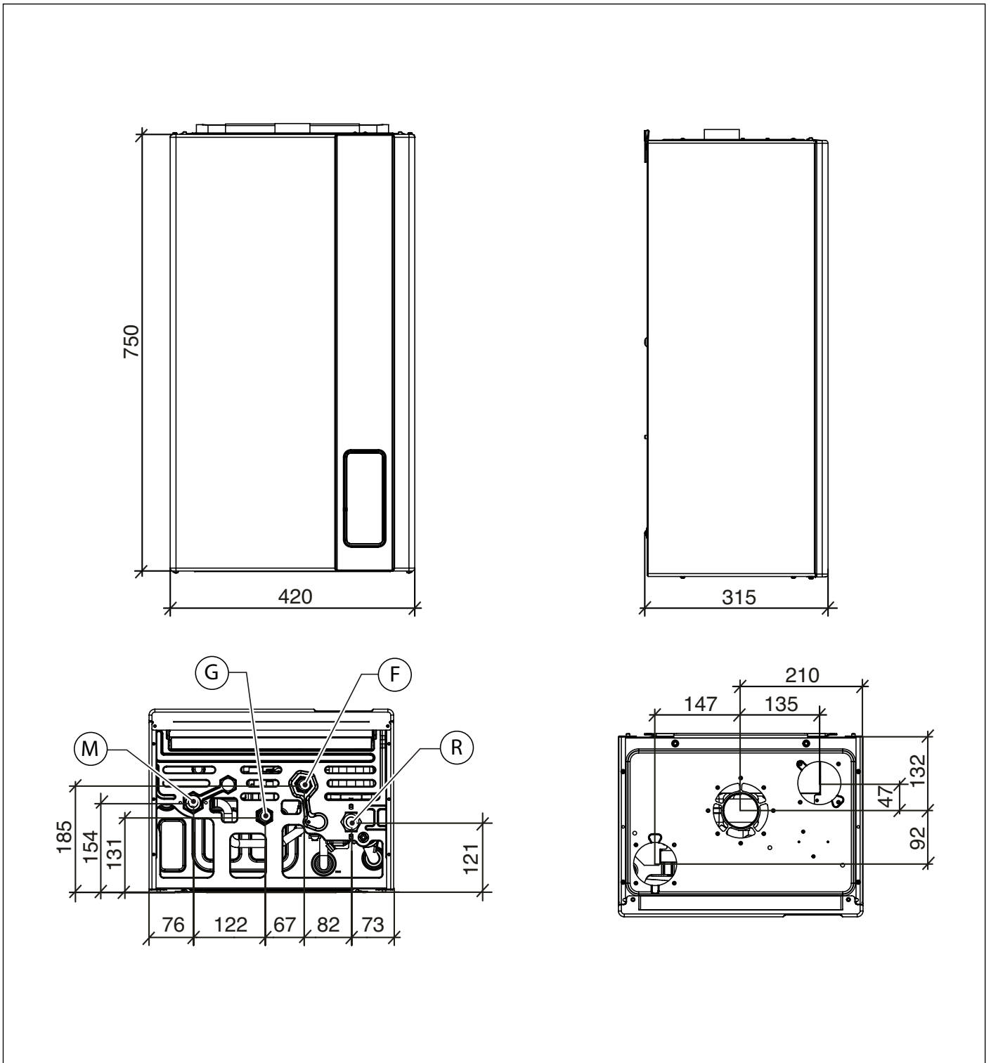
Рис. 4 Габарити RTFS
