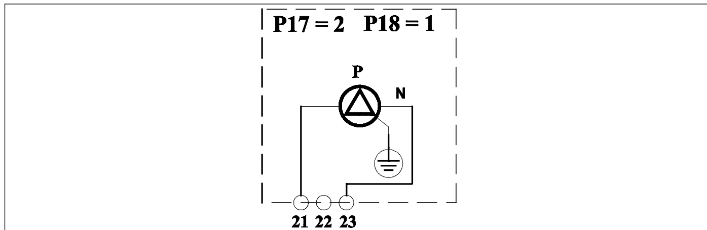
Рис. 27 Схема підключення багатofункційного реле
