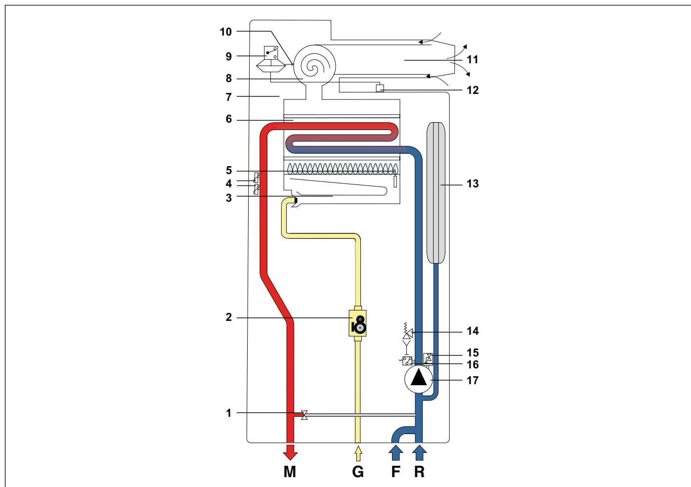
Рис. 6 Схеми гідравлічних підключень RTFS
