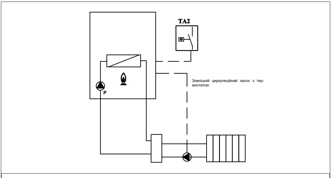
Рис. 33 Робота реле по зовнішньому запросу
