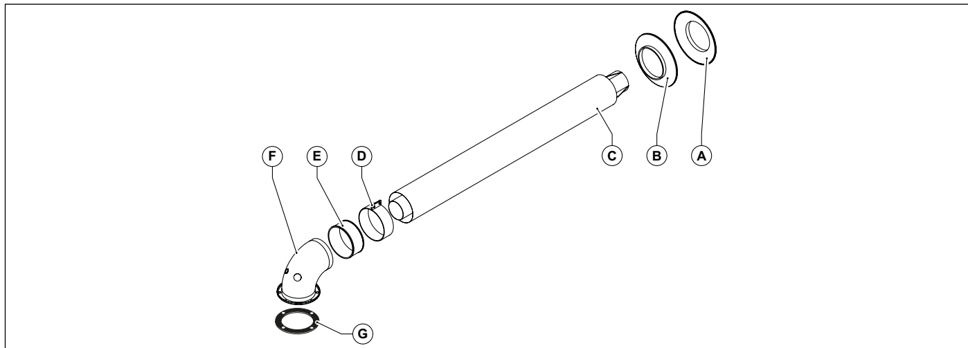
Рис. 10 Коаксиальний комплект OKITCONC00
