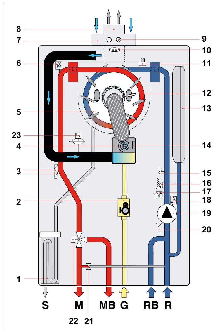
Рис. 8 Гідравлична схема моделі KRB
