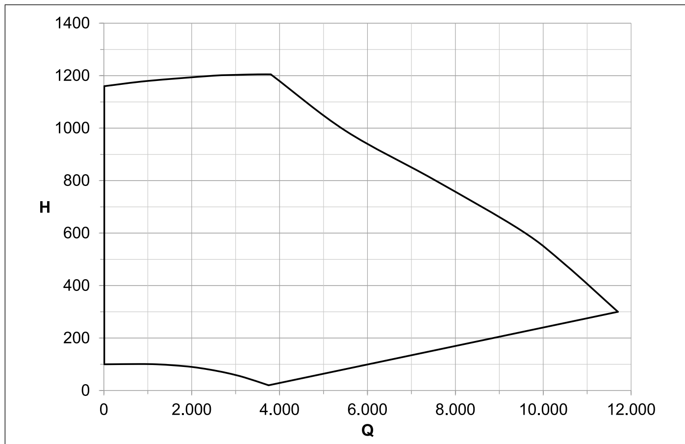
Рис. 20 Наявний напір YONOS PARA HF 25/12
