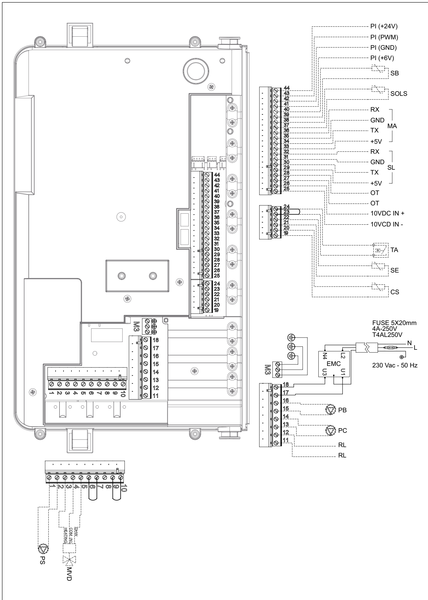
Рис. 27 Усі підключення виконуються монтажником
