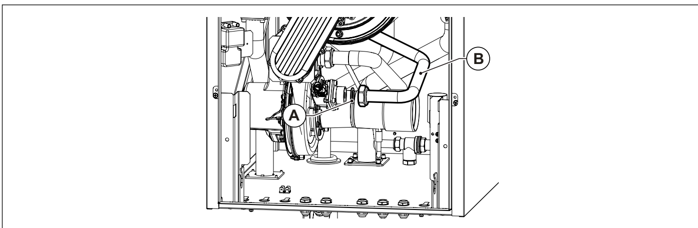
Рис. 30 Замініть діафрагму газу
