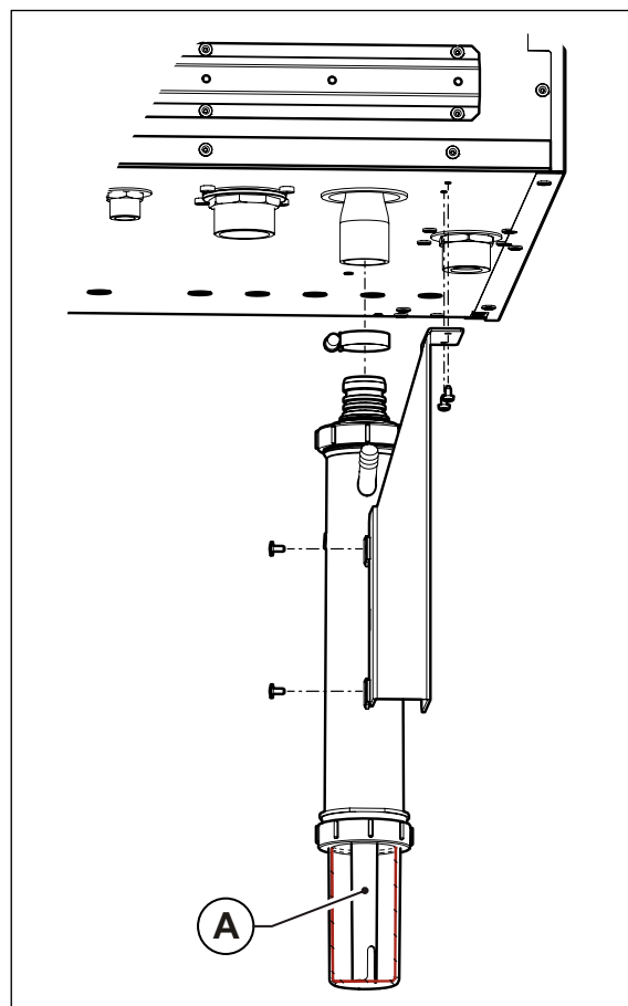
Рис. 8 Закріплення збірника
