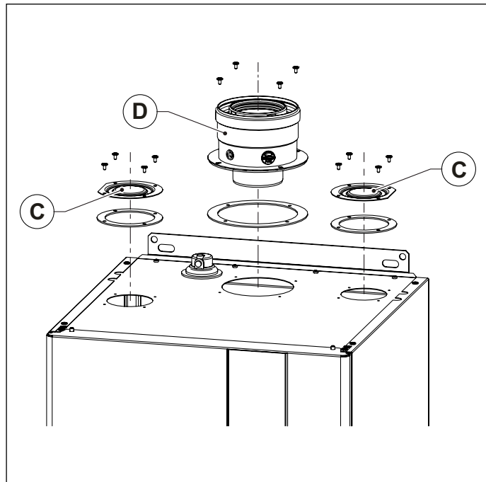
Рис. 10 Установка коаксіального набору
