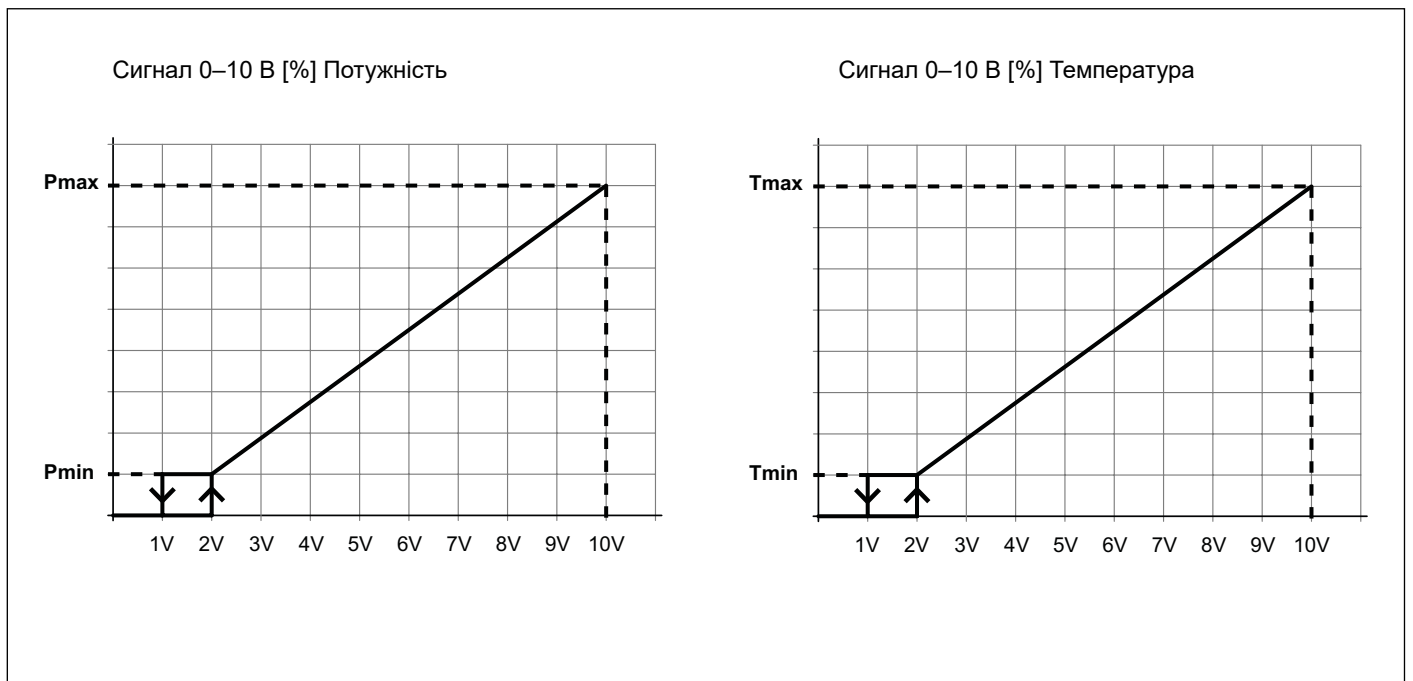
Рис. 18 Сигнал 0–10 В постійного струму
