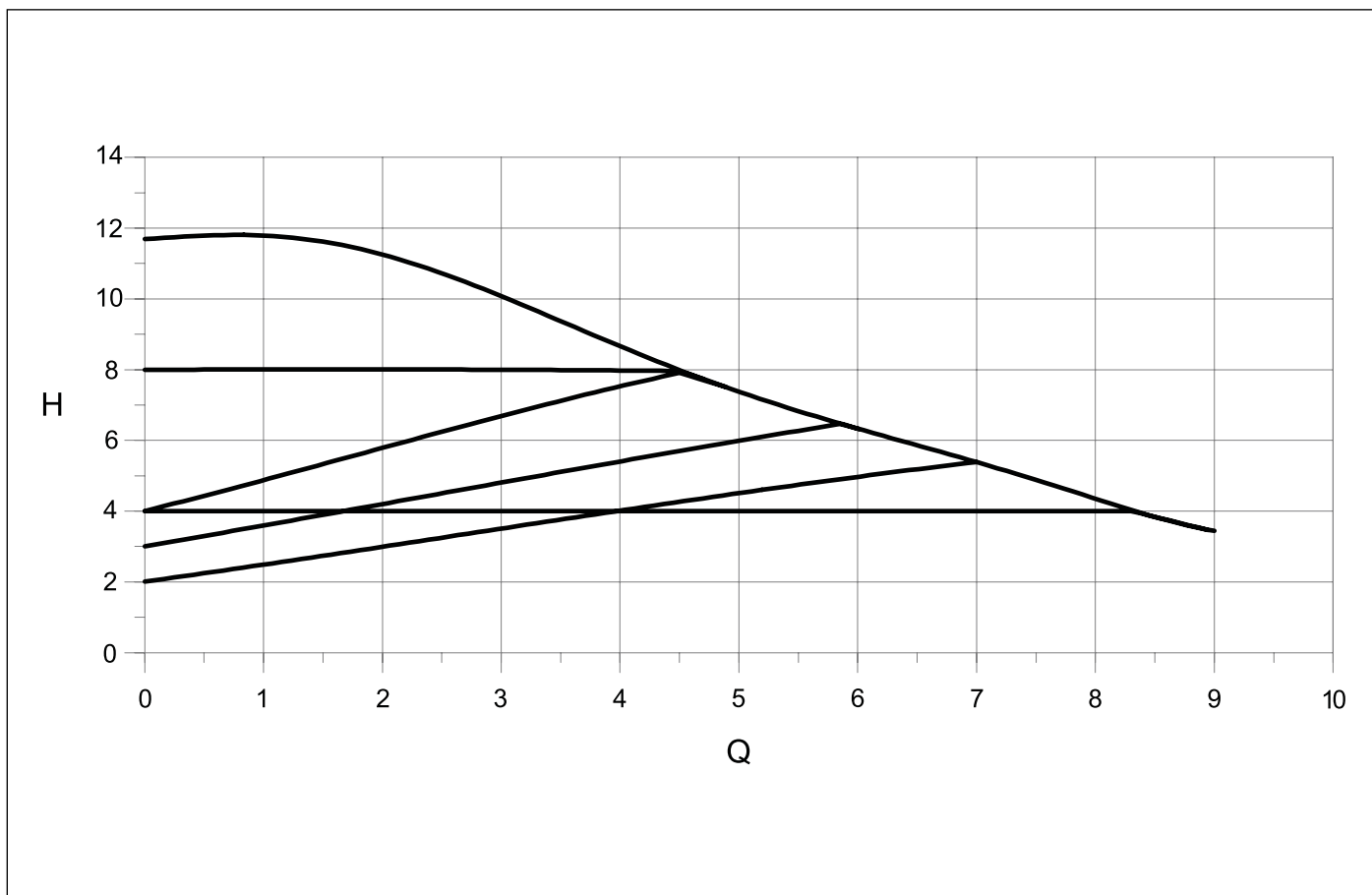
Рис. 22 Наявний напір UPMXXL 25 - 120 - 180 AUTO
