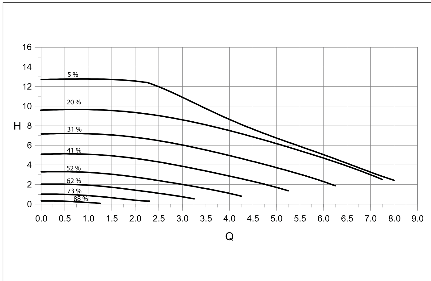
Рис. 21 Наявний напір UPMXL 25 - 125 - 180 PWM
