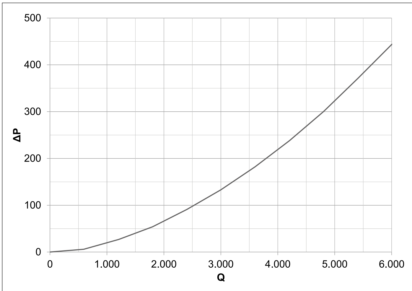
Рис. 19 Гідравлічний опір
