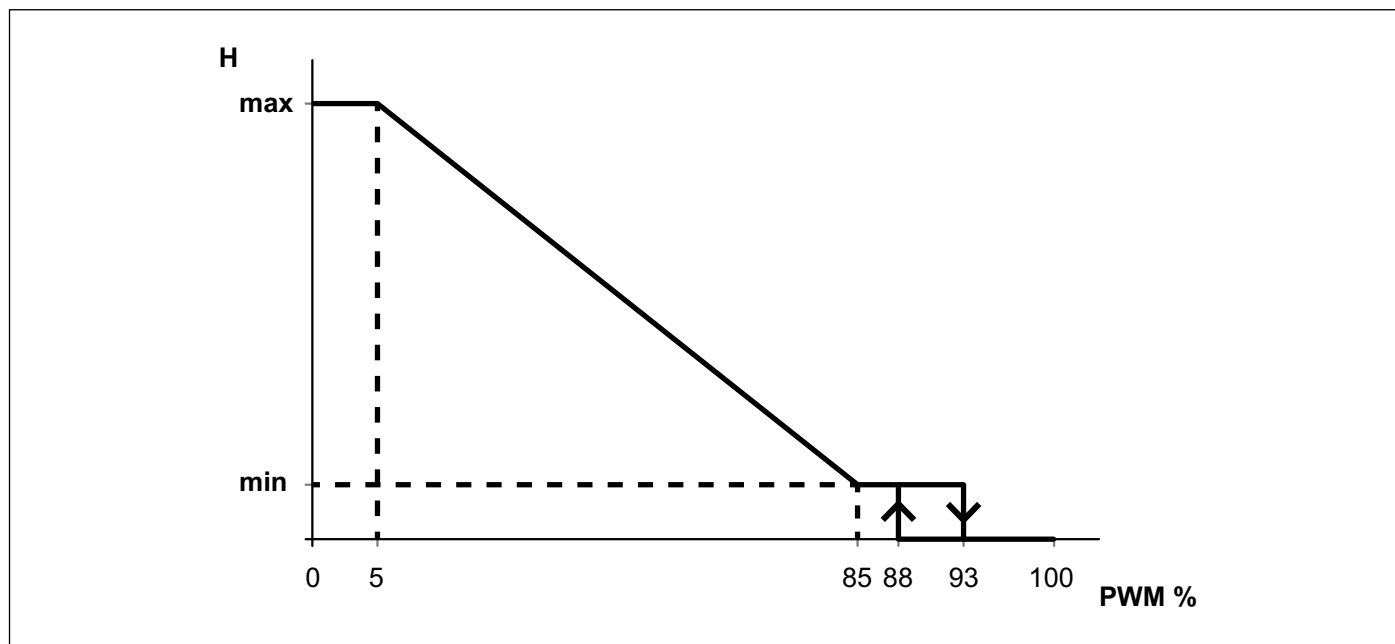
Рис. 23 Сигнал ШІМ
