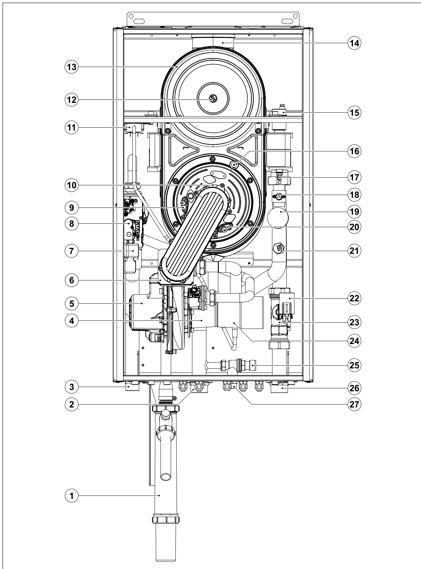
Рис. 4 Компоненти (I)
