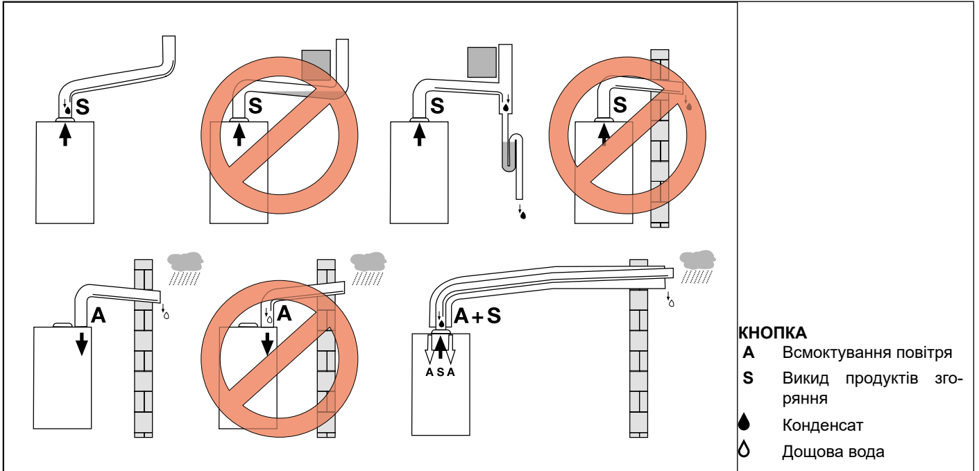
Рис. 11 Приклади монтажу
