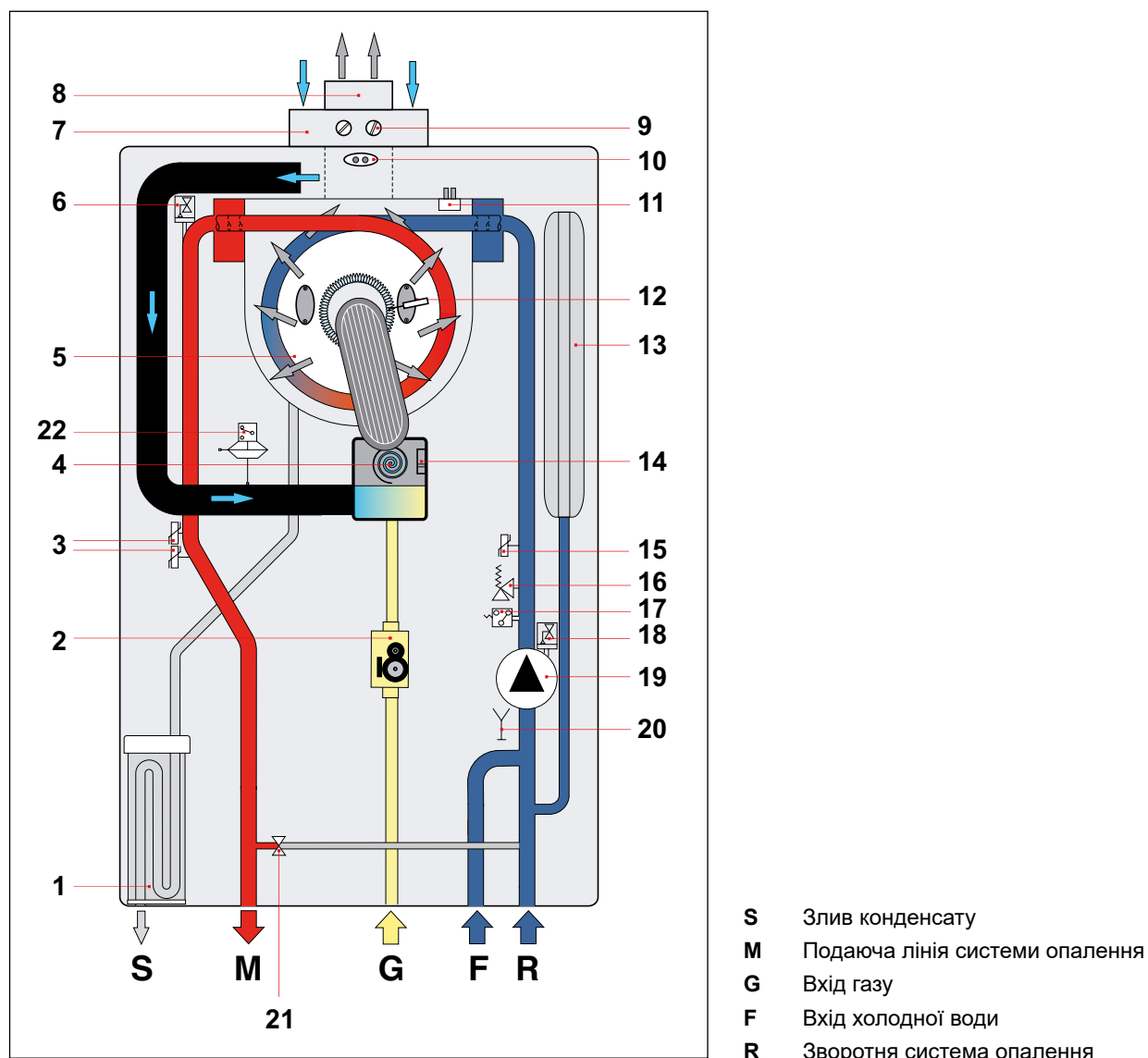
Рис. 7 Гідравлячна схема моделі KR
