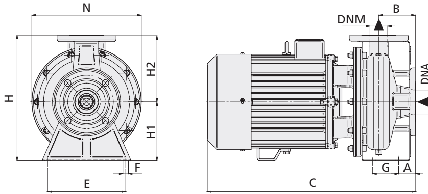
Flange Flanges
