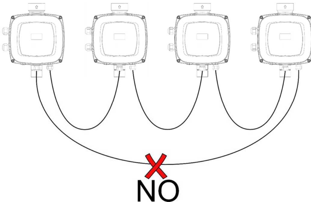
Kuva 5: Älä tee silmukkakytkentöjä
