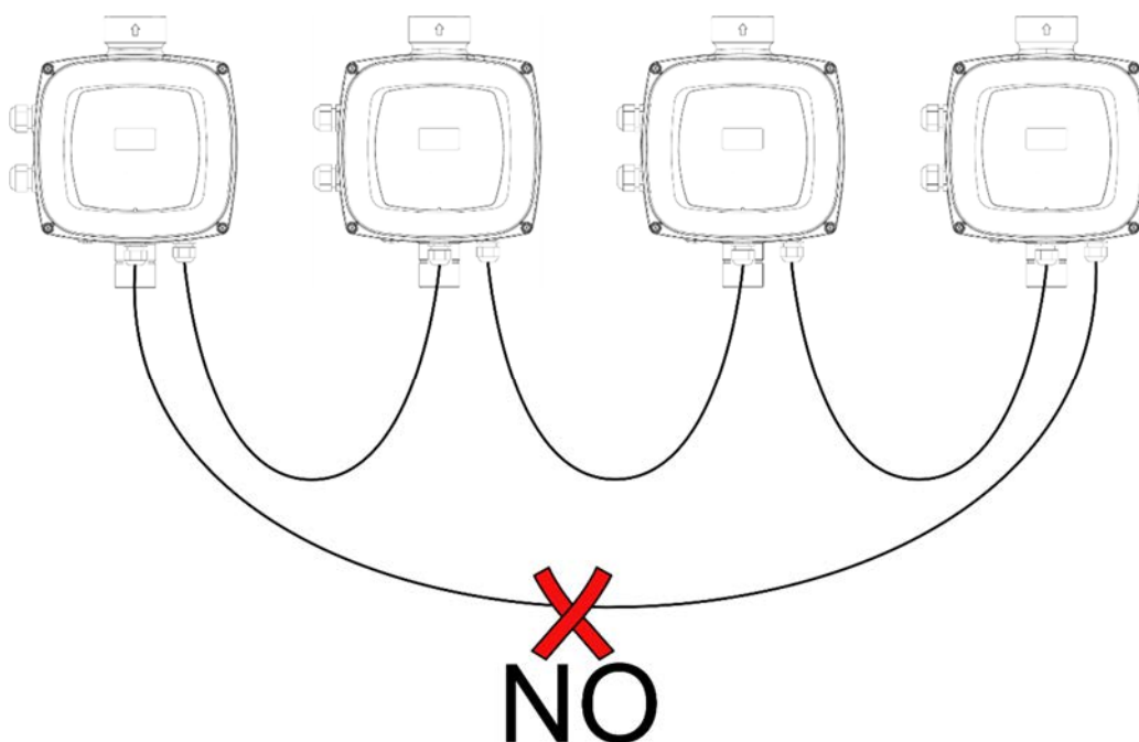
Obrázok 5: Nevykonávať prstencové spojenia
