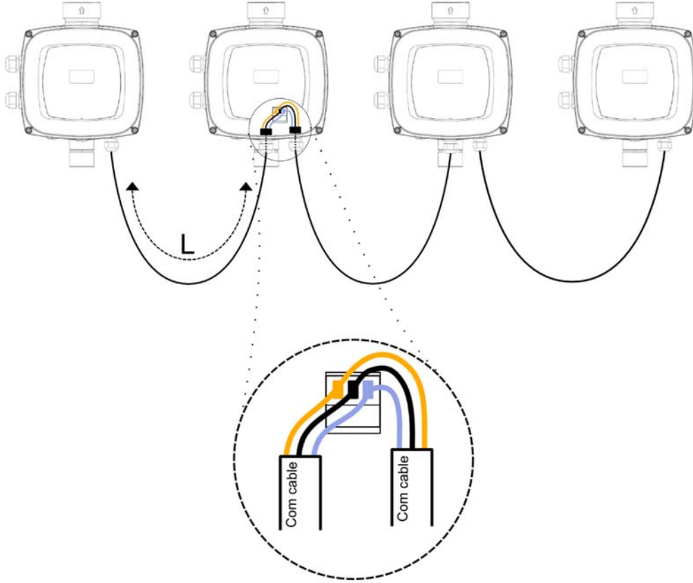
Şekil 4: 4 aygıtlı multi inverter haberleşmenin bağlantı örneği
