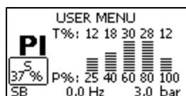
Рисунок 13: Гистограмма мощности
