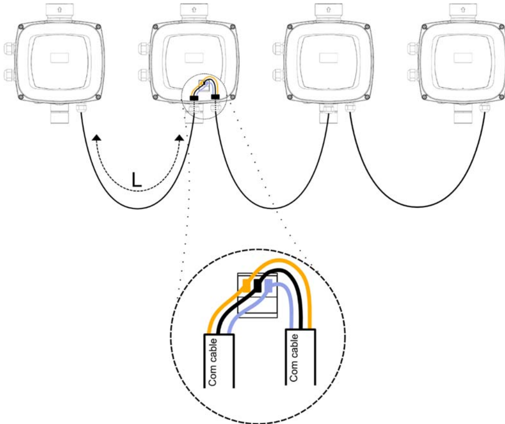
Figura 4: Exemplo de ligação da comunicação multi inversor com 4 dispositivos
