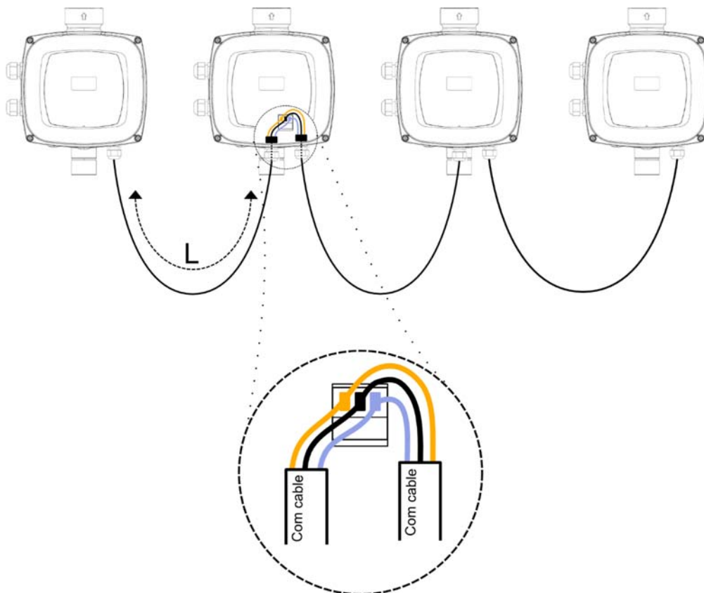
Rysunek 4: Przykład połączenia komunikacji multi inwerter z 4 urządzeniami
