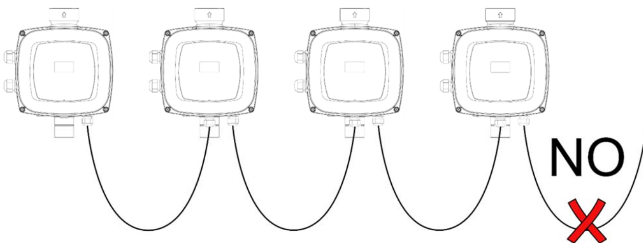
Σχήμα 7: Μην αφήνετε καλώδια συνδεδεμένα μόνο στο ένα άκρο
