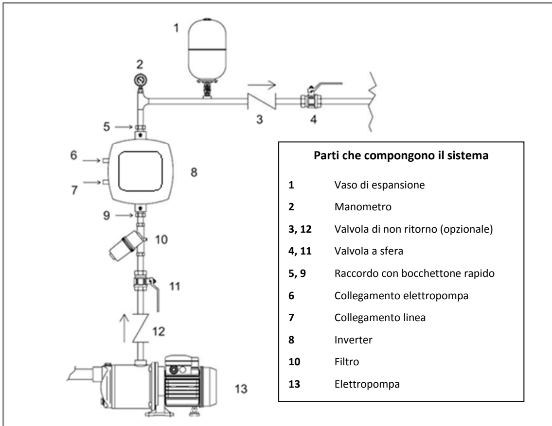
Figura 1: Installazione idraulica
