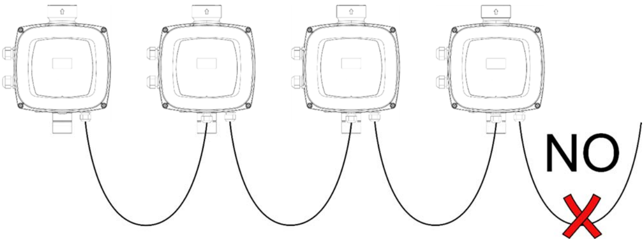
Малюнок 7: Не залишайте кабелі під'єднаними лише за один кінець
