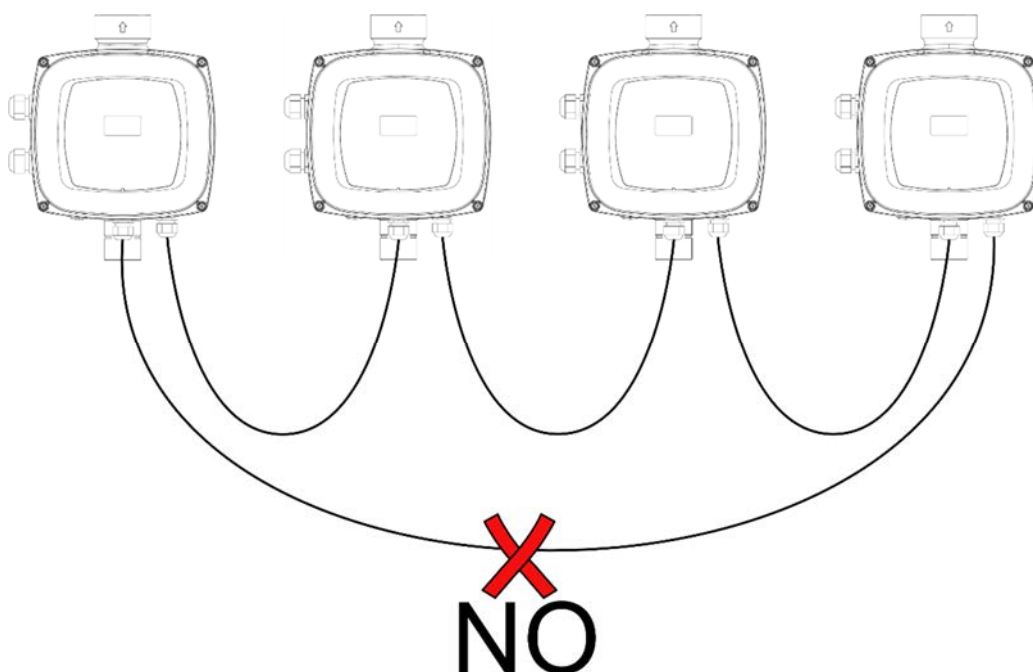
Rysunek 5: Nie wykonywać połączenia na pierścień
