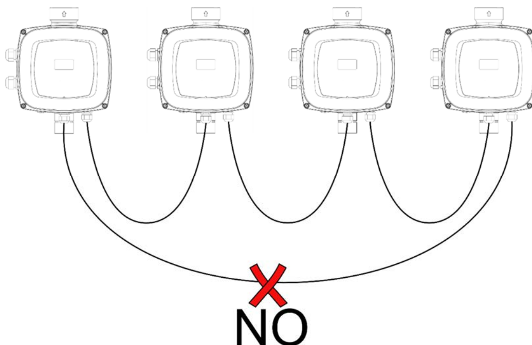
Figura 5: Non eseguire connessioni ad anello
