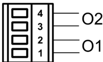
Рисунок 3: Соединение выходов
