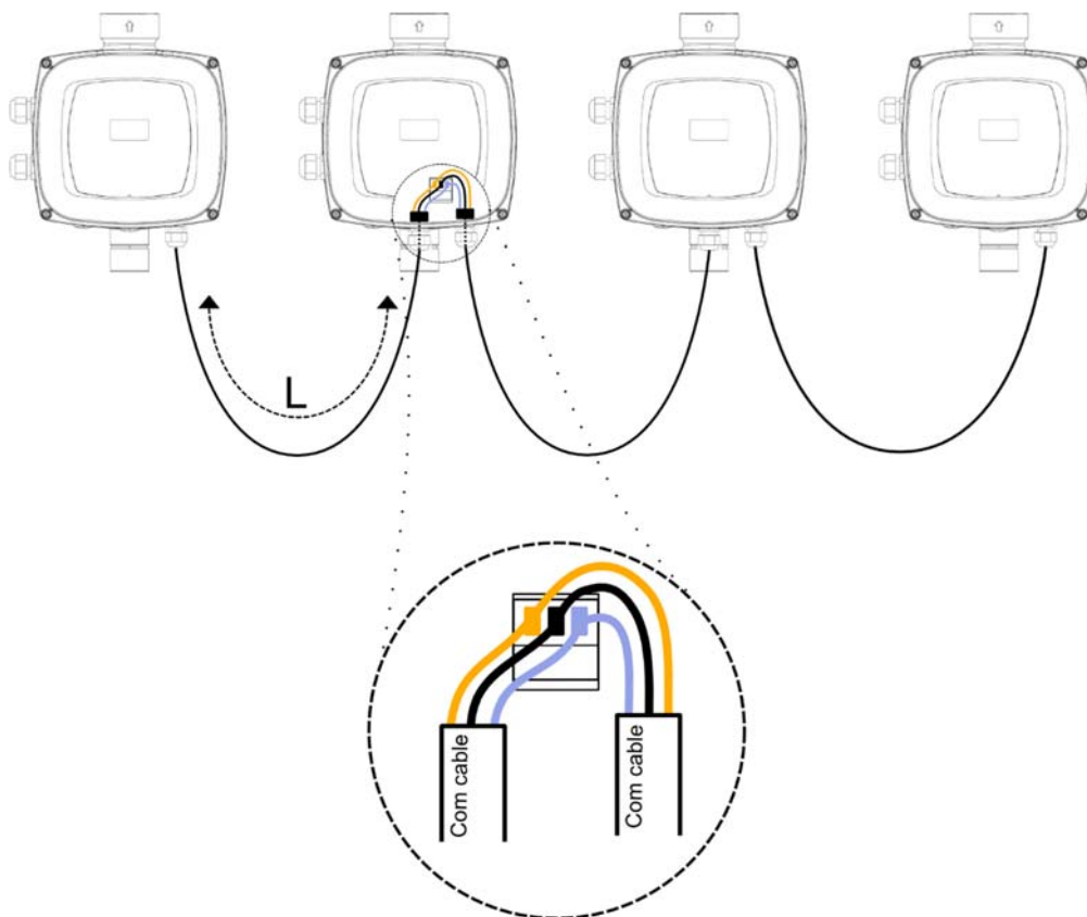
Obrázok 4: Príklad pripojenia komunikácie pre multi inverter so 4 zariadeniami
