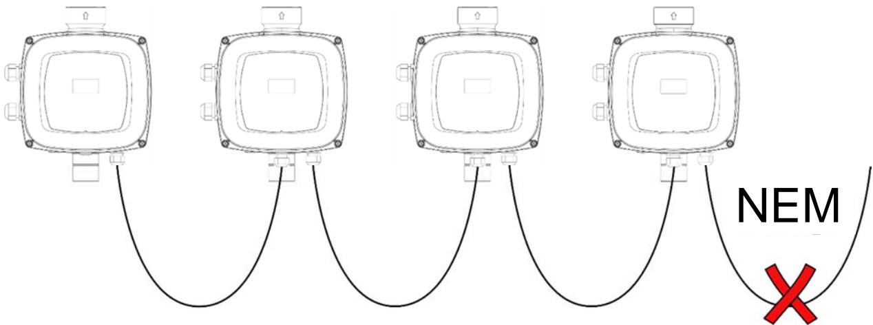
7. Ábra: Ne hagyjon egyoldalon bekötött kábelt a rendszerben
