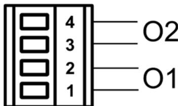
Kuva 3: Lähtöliitäntä
