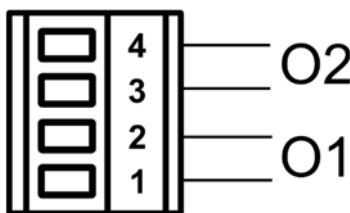
3. Ábra: A kimenetek bekötése
