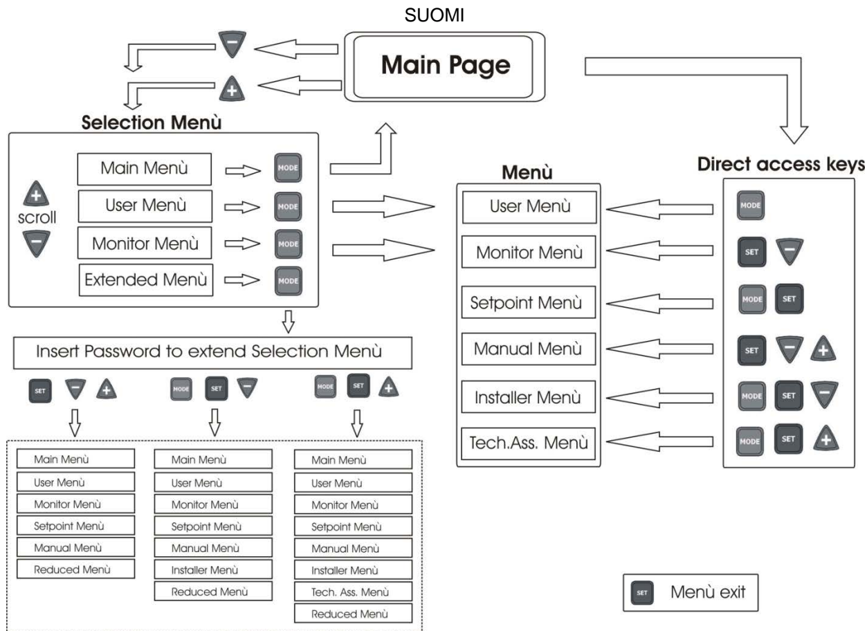
Kuva 11: Valikoiden avauskaavio
