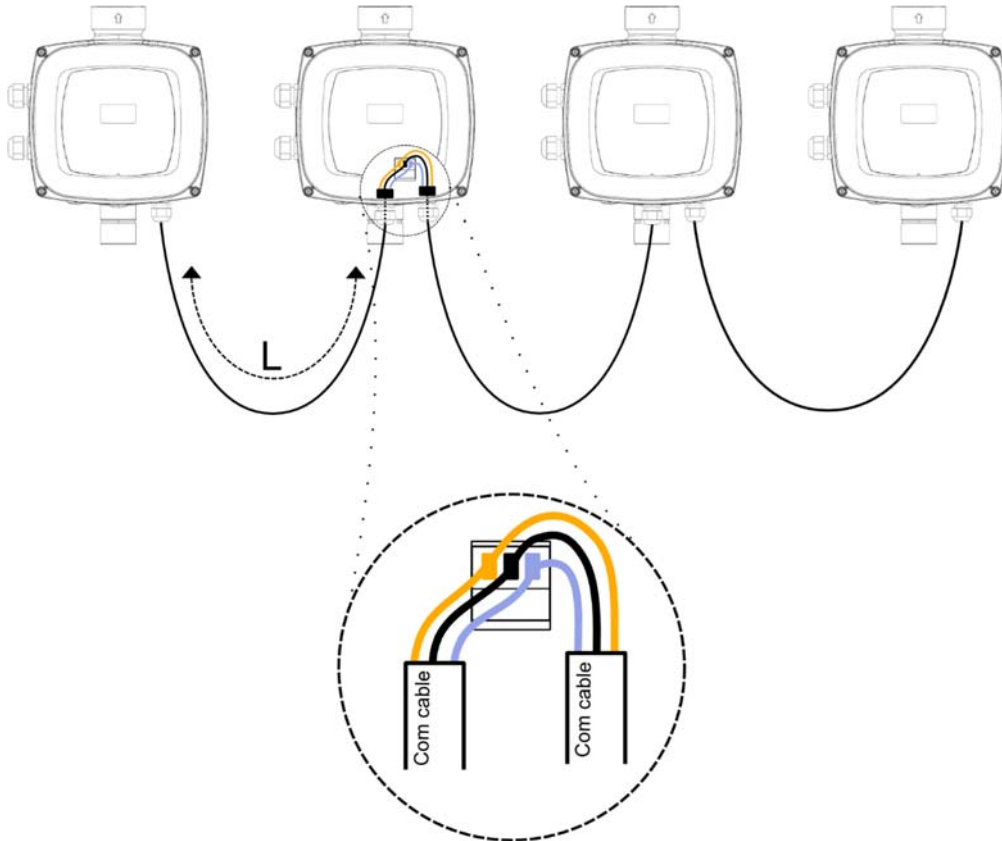
Figura 4: Exemplu de conexiune a comunicării multi inverter cu 4 dispozitive
