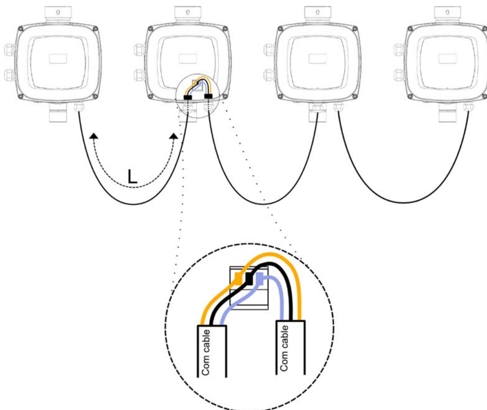
Abbildung 4: Beispiel für den Anschluss der Kommunikation Multi-Inverter mit 4 Geräten
