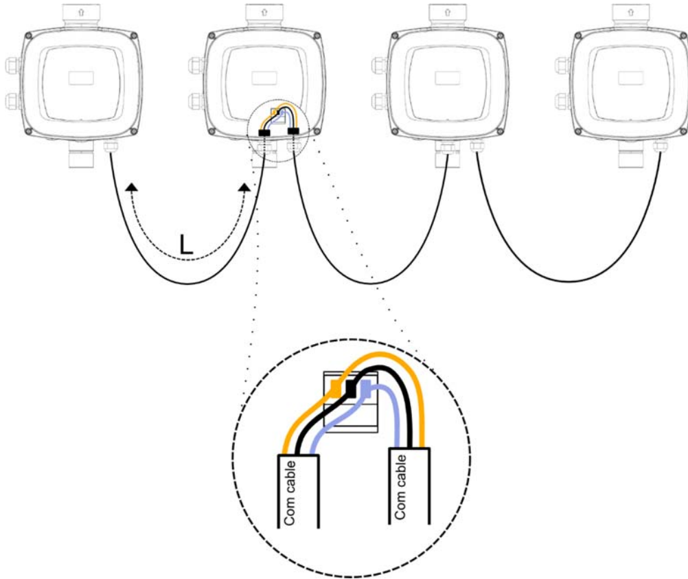
Малюнок 4: Приклад під'єднання мультіінвертора до 4 пристроїв
