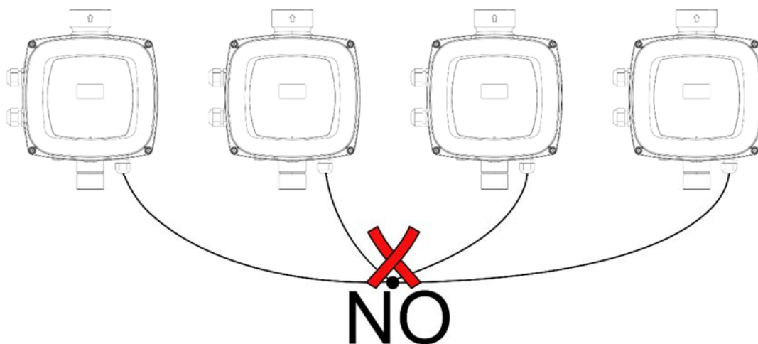
Figura 6: Non eseguire connessioni a stella
