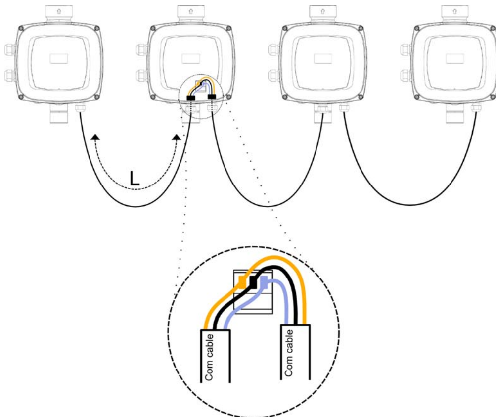
4. Ábra: Példa multi inverteres kommunikációs összekötésre 4 db.berendezéshez
