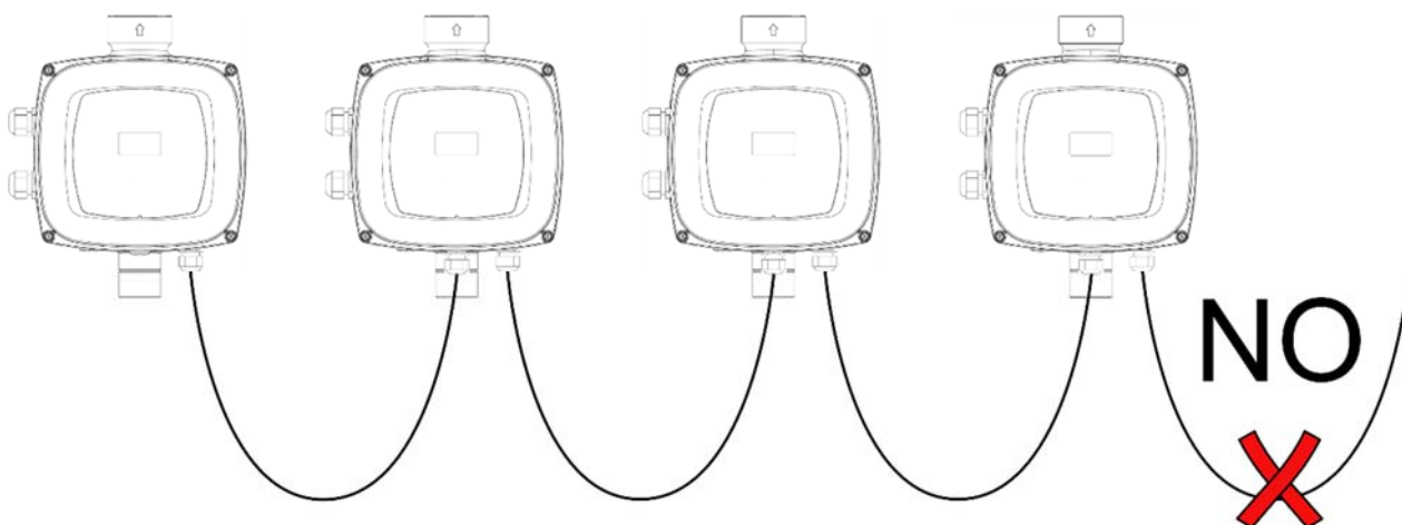
Kuva 7: Älä jätä johtoja kytketyiksi ainoastaan yhdestä päästä
