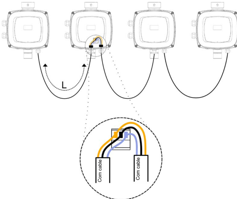
Fig. 4: Exempel på anslutning för kommunikation mellan flera inverterar med fyra anordningar
