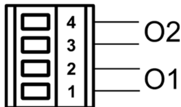
Obrázok 3: pripojenie výstupov
