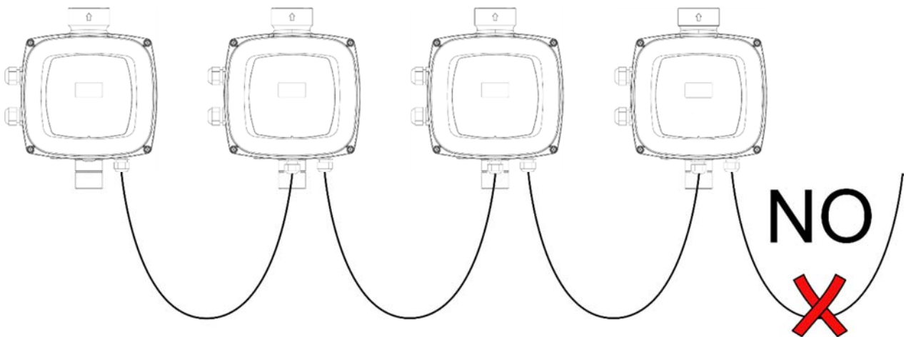
Abbildung 7: Keine nur an einem Ende angeschlossenen Kabel belassen
