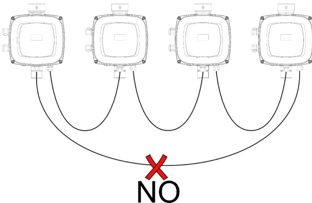
Σχήμα 5: Μην κάνετε σύνδεση δακτυλίου
