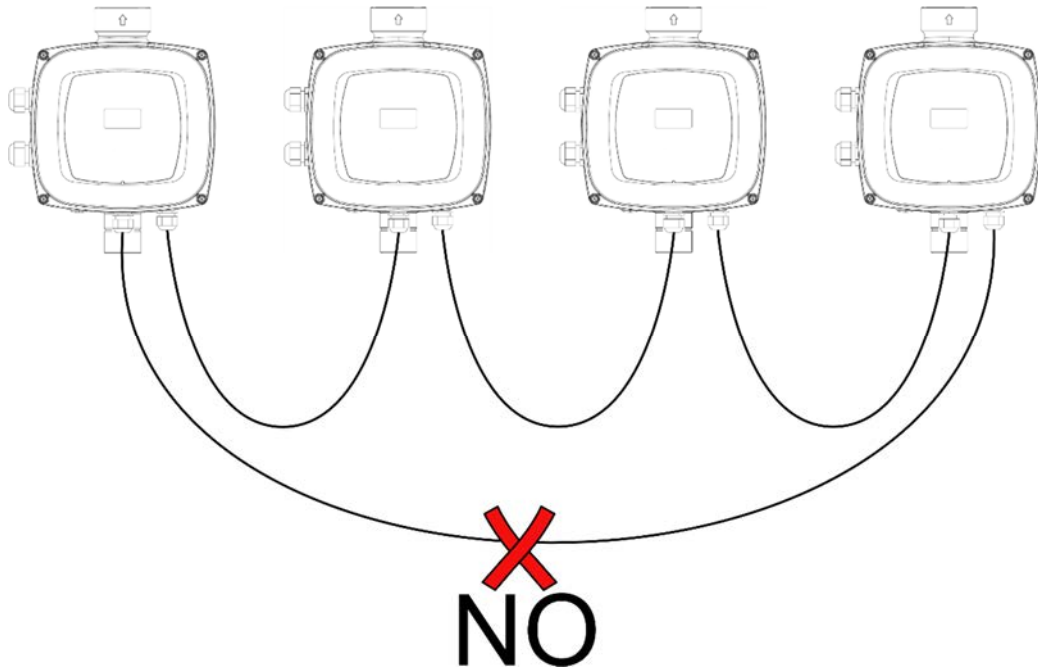
Abbildung 5: Keine Schleifenschaltung herstellen
