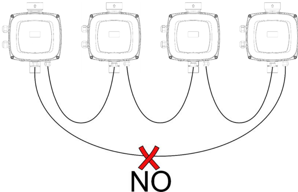
Şekil 5: Halka bağlantılar gerçekleştirilmeyiniz
