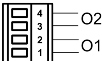
Figura 3: Conexiune ieșiri
