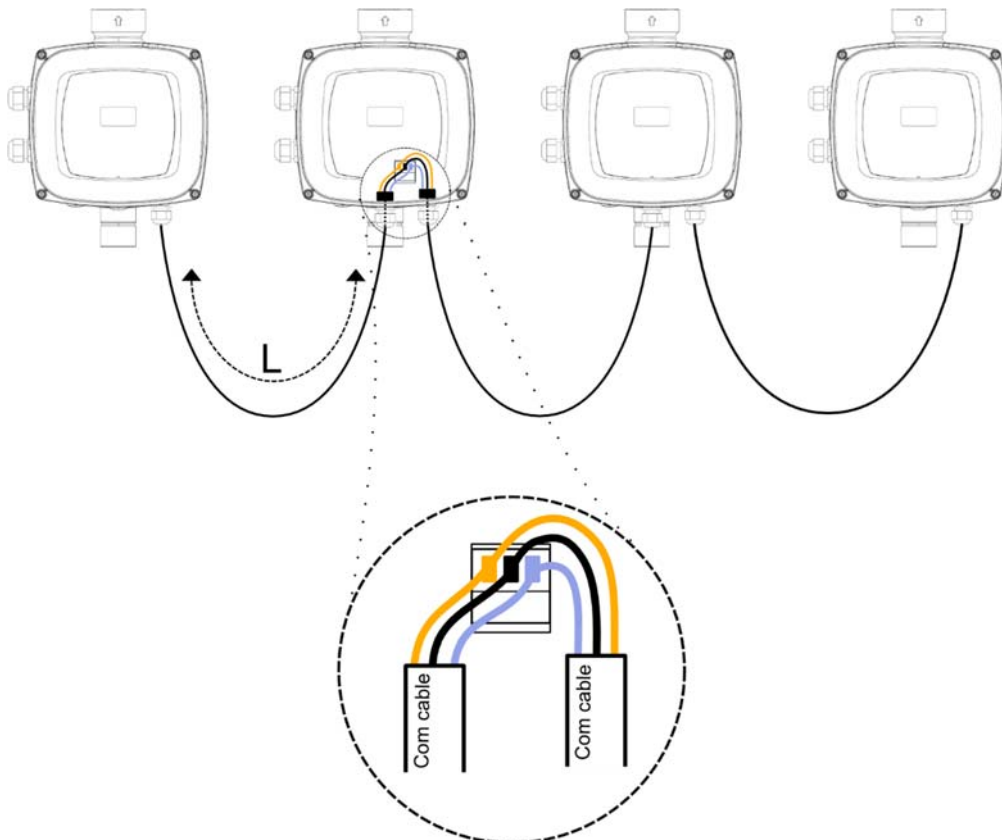
Рисунок 4: Пример соединения коммуникации мульти-инвертора с 4 устройствам
