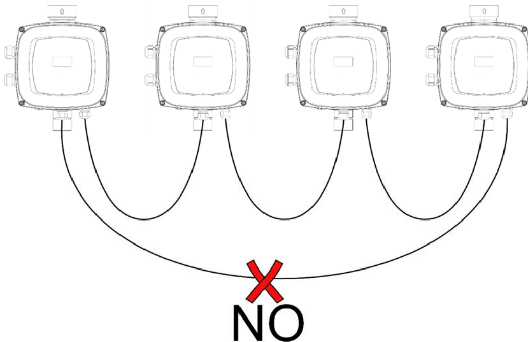
Малюнок 5: Не під'єднуйте кабелі за кільцевою схемою
