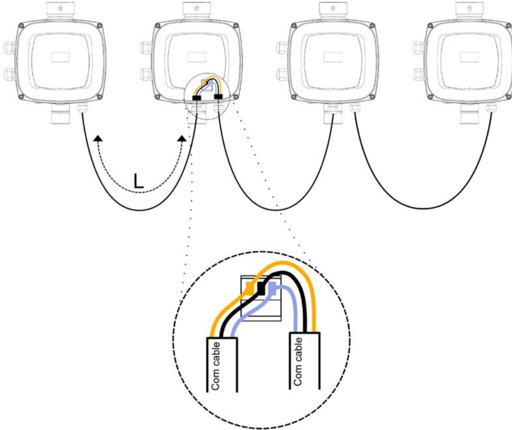
Figura 4: Ejemplo de conexión de la comunicación multi inverter con 4 dispositivos
