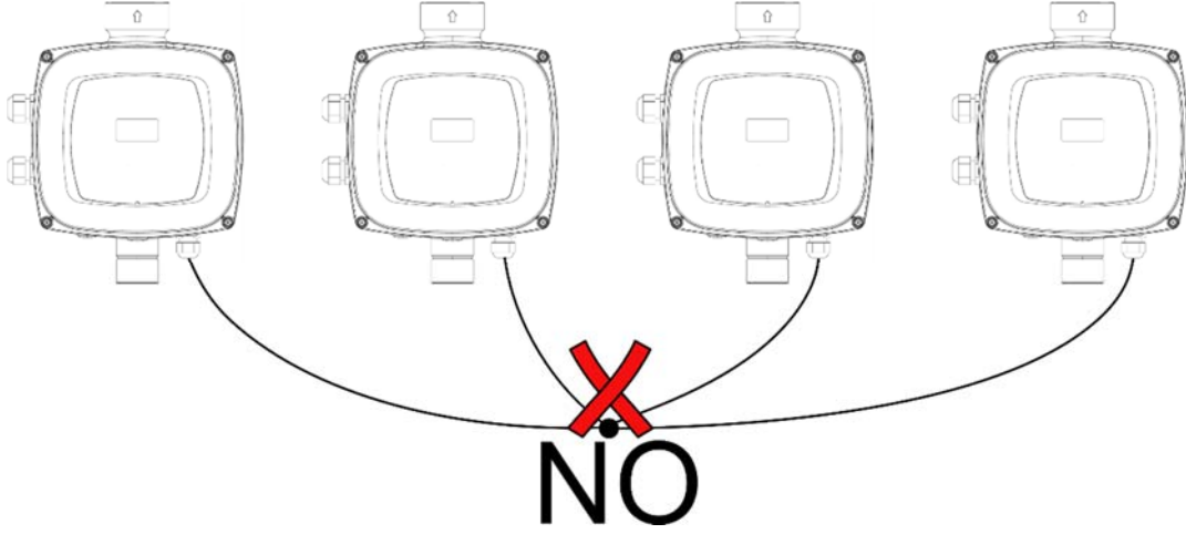
Şekil 6: Yıldız bağlantılar gerçekleştirilmeyiniz
