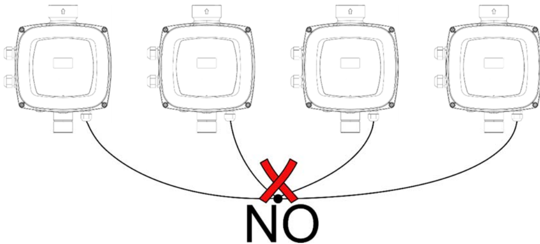
Abbildung 6: Keine Sternschaltung herstellen
