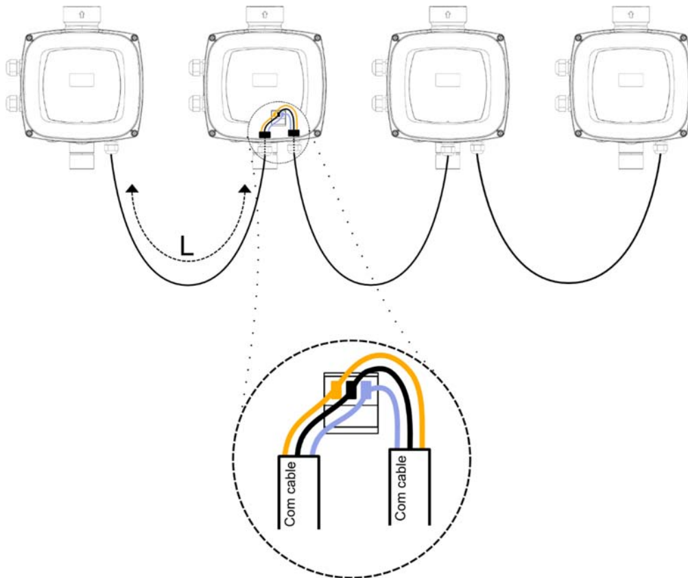
Obr. 4: Příklad připojení komunikace multi inverter se 4 zařízeními
