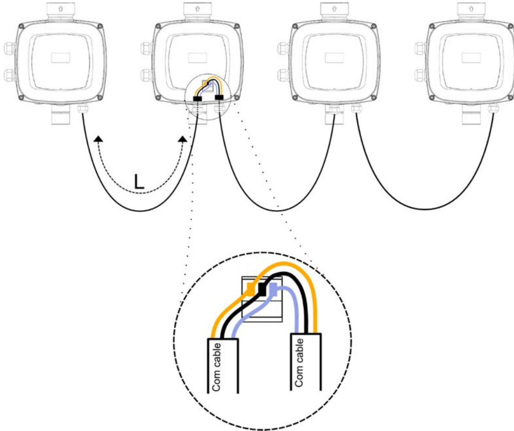
Kuva 4: Esimerkki 4 laitteen moni-invertterijärjestelmän yhteyskytkennästä
