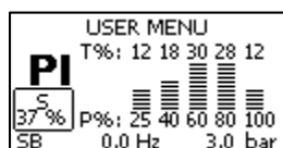
Obr. 13: Sloupcový diagram výkonu
