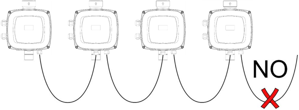
Şekil 7: Tek bir uca bağlanmış kablolar bırakmayınız
