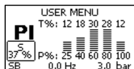
Малюнок 13: Гістограма потужності
