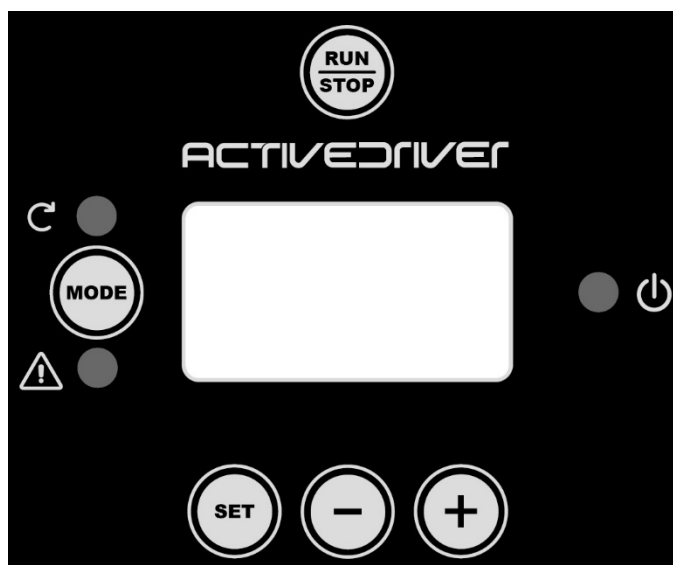
Fig. 9: Gränssnittets utseende
