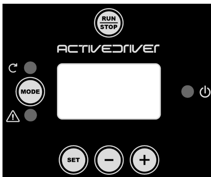
Kuva 9: Käyttöliittymän ulkomuoto
