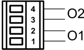
Şekil 3: Çıkışların bağlantısı
