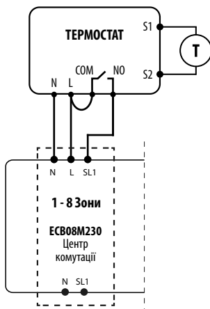
в) Схема підключення до центру комутації
