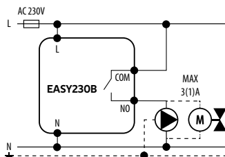
б) Схема підключення до котла
