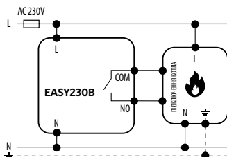
а) Схема підключення до котла
