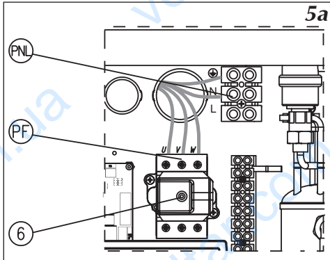
Рис.5а Подключение котла ЕКО.М1 в однофазную электрическую сеть.
