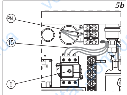
Рис.5б Подключение котла ЕКО.М1 в трехфазную электрическую сеть (касается котлов 4 кВт, 6 кВт и 8 кВт).
