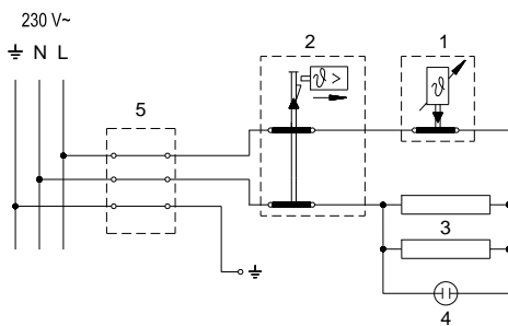
Електросхема
