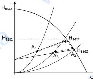
Рис. 9 "АВТО ADAPT "
