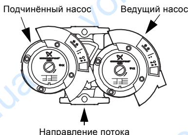
Рис. 17 Ведущий/подчинённый насосы
