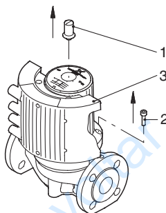
Рис. 1 Снятие блока управления
