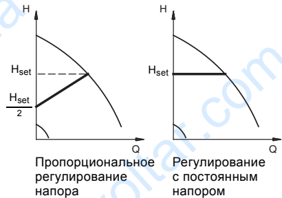
Рис. 10 Регулирование напора
