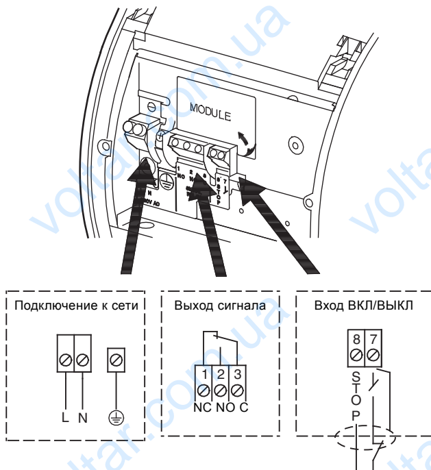
Рис. 7 Схема электрических соединений
