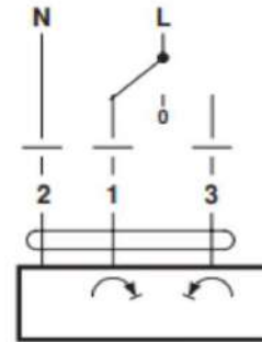
Схема підключення приводу
