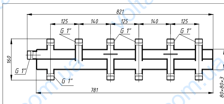
Колектор K51B.125M
