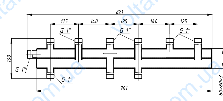
Колектор K51B.125M
