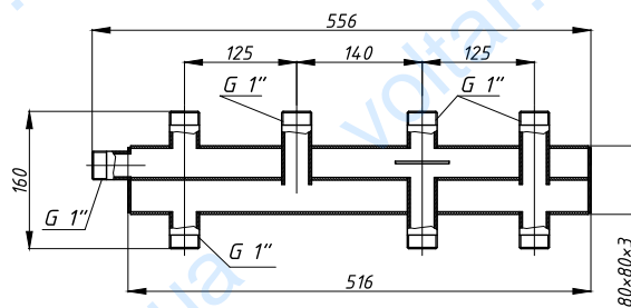
Колектор K31B.125M
