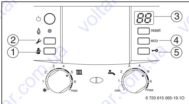
Рис 36 Элементы управления
