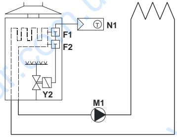
Прямое управление газовым настенным котлом
