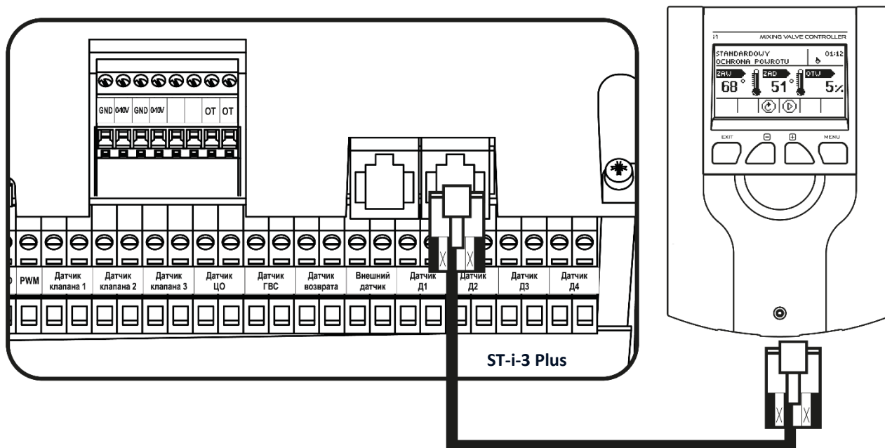
Примерное соединение дополнительного клапана с главным контроллером ST-i-3 Plus OT
