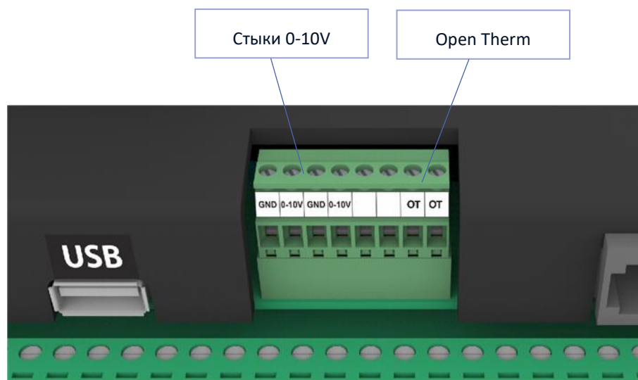
Соединитель стыков с напряжением 0-10 V
