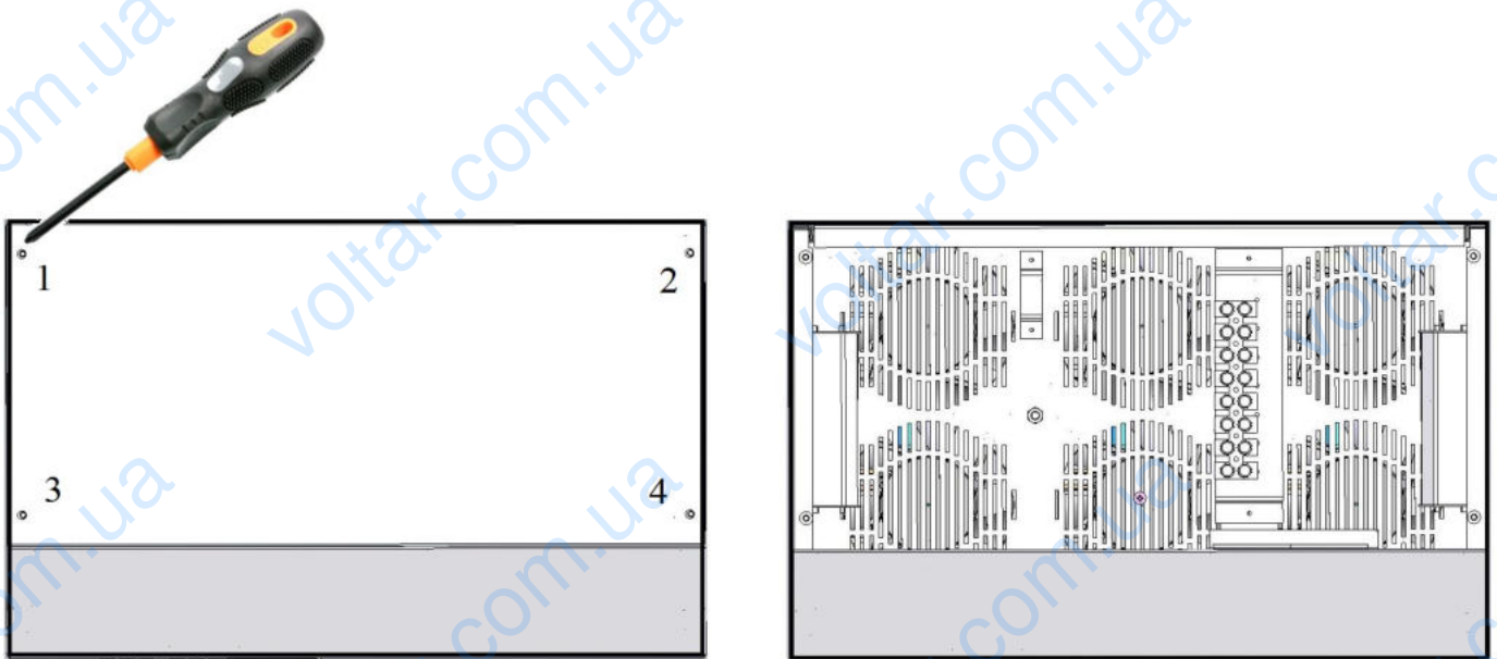
Рисунок 6. Схема зняття захисної кришки зверху корпусу стабілізатора
