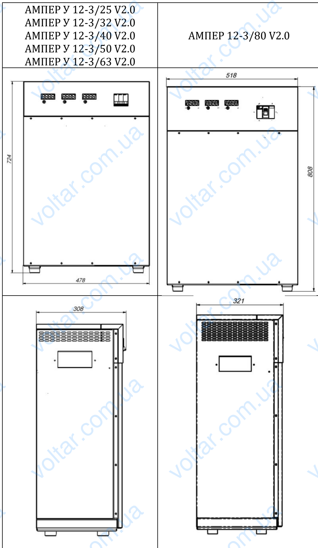
Рисунок 4. Габаритні розміри стабілізаторів
