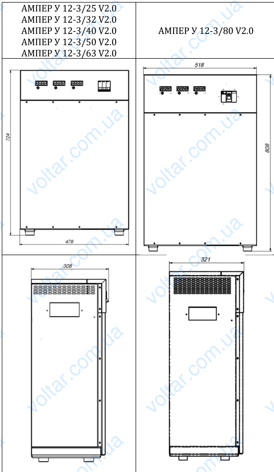
Рисунок 4. Габаритные размеры стабилизаторов
