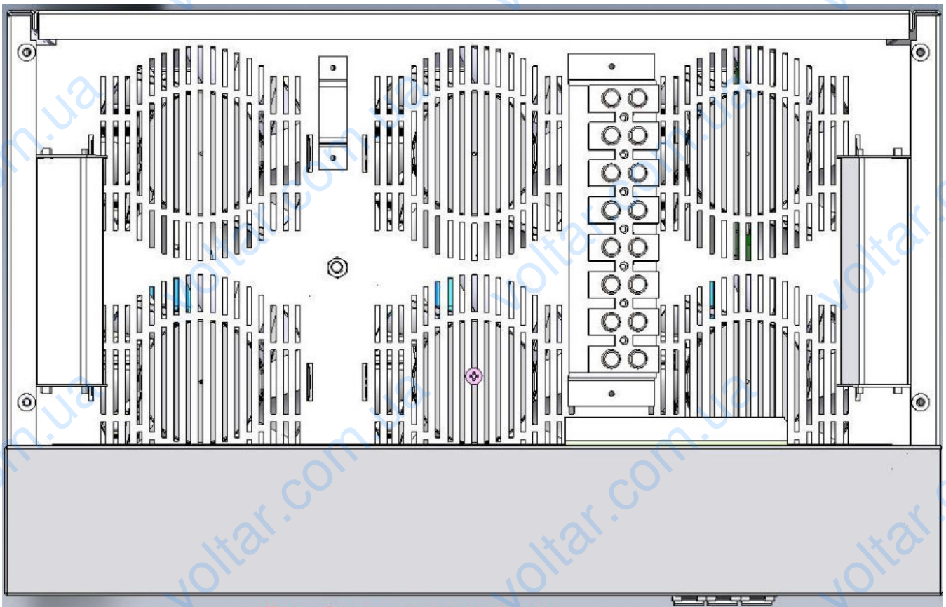
Рисунок 3. Внешний вид верхней части стабилизатора
