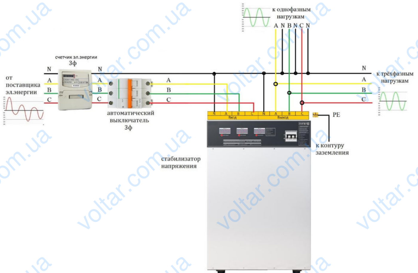
Рисунок 5. Схема подключения стабилизатора к трёхфазной сети
