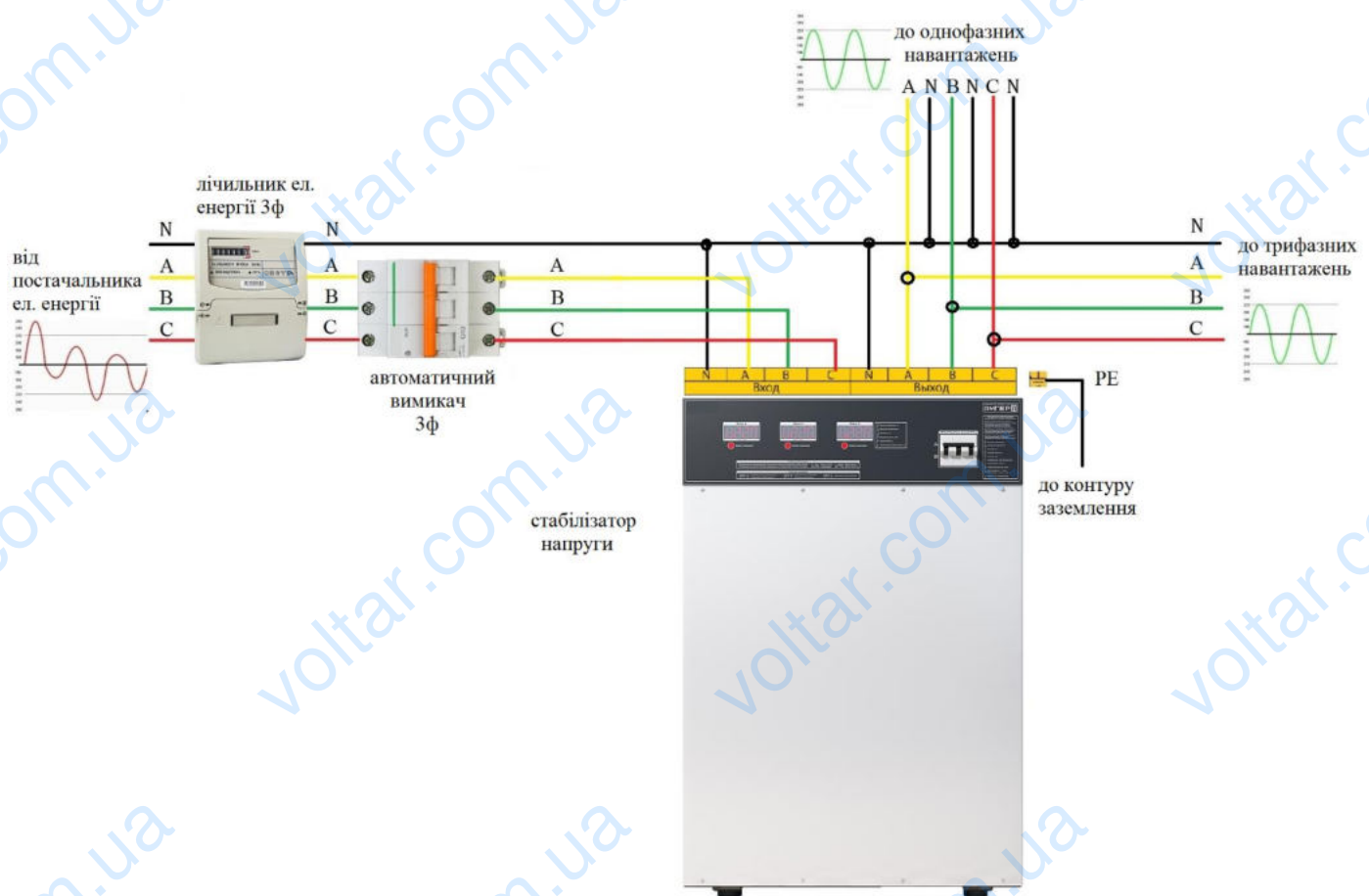
Рисунок 5. Схема підключення стабілізатора до трифазної мережі
