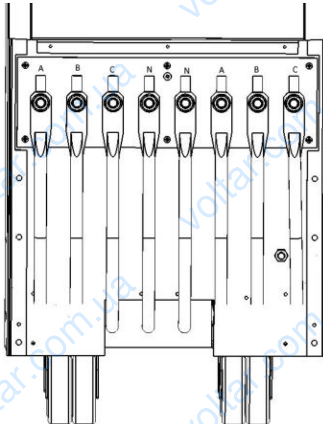
Рисунок 6. Внешний вид передней части стабилизатора Герц-ПРО на 100-160А
