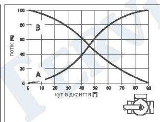
Характеристика клапану
