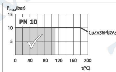
Діаграма тиск-температура
